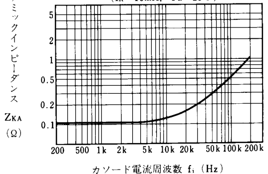
ダイナミックインピーダンス 対カソード電流周波数特性 ( I_K = 10\text{mA} , T_a = 25^\circ\text{C} )
