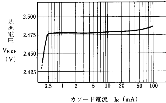
基準電圧対カソード電流特性例 ( V_{KA} = V_{REF} , T_a = 25^\circ\text{C} )
